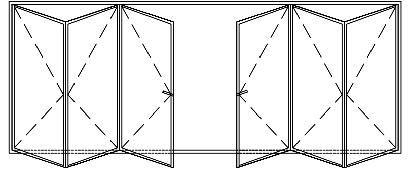
3 + 3 PANEL STACK DOOR NTS
